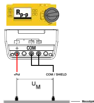
Messung: R_{p\text{-p}} Punkt-zu-Punkt Widerstand
