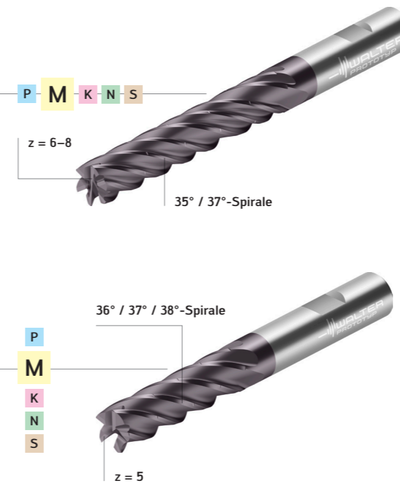
Vollhartmetallfräser Xill-tec® MC233 Advance
