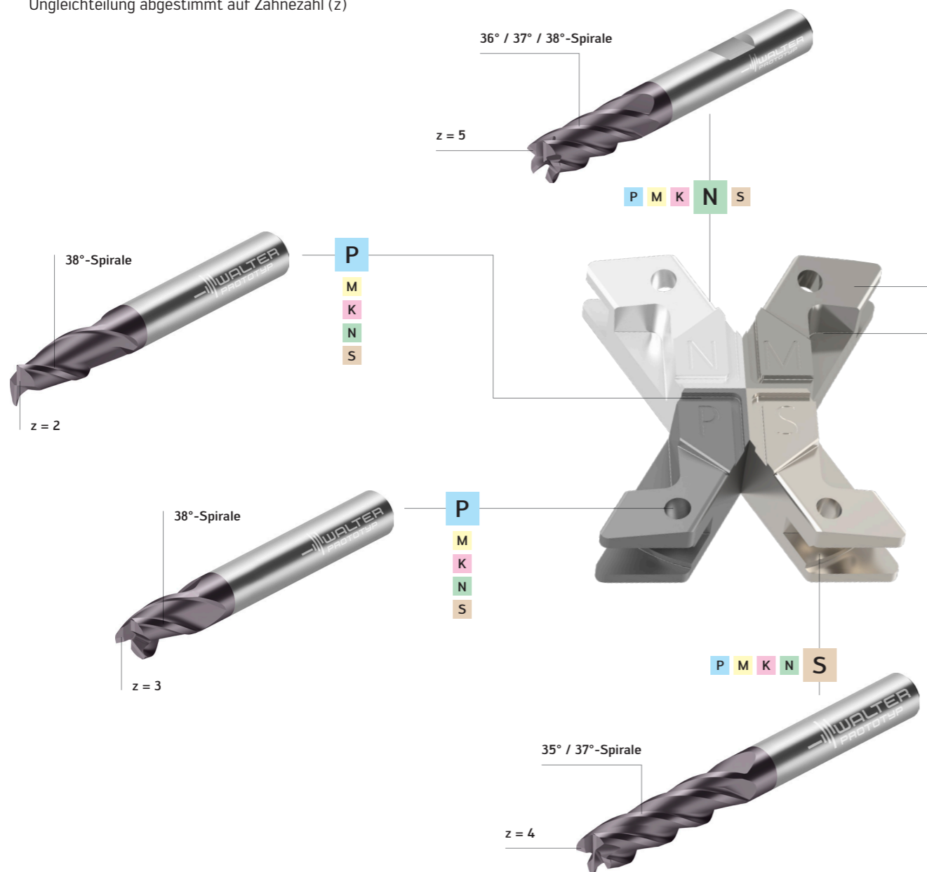
Vollhartmetallfräser Xill-tec® MC230 Advance
